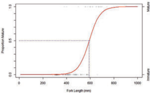
Рисунок 6. Огива созревания самок азиатского стрелозубого палтуса по длине Figure 6. The length of maturation of female Asian arrowtooth halibut
