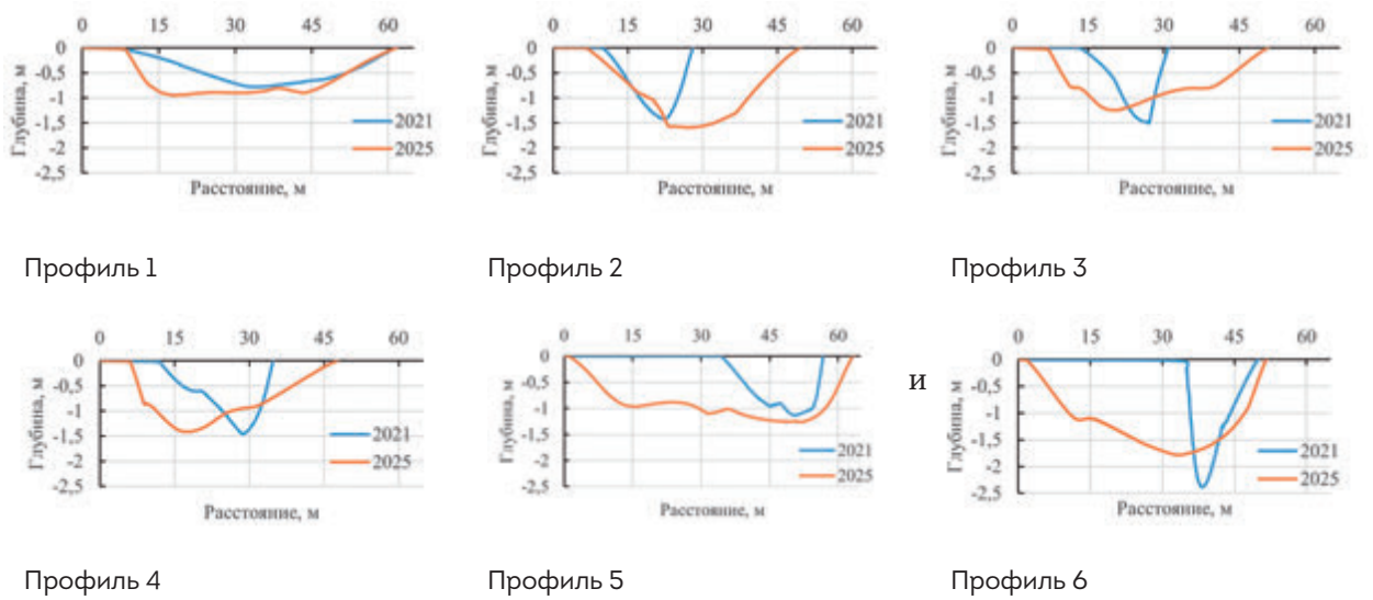
Рисунок 4. Поперечные профили русла р. Промысловая в шести репрезентативных створах, по данным батиметрических съемок 2021 и 2025 годов Figure 4. Cross-sectional profiles of the Promyslovaya River bed at six representative cross-sections based on bathymetric surveys from 2021 and 2025
