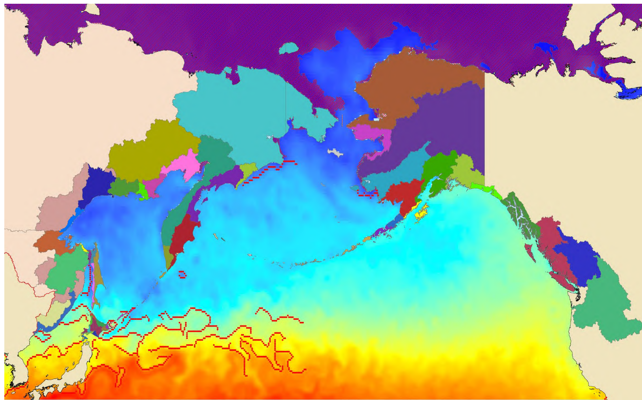
Фронтальные зоны (градиент 1^{\circ}\text{C} и более) на 09 ноября 2025 года
