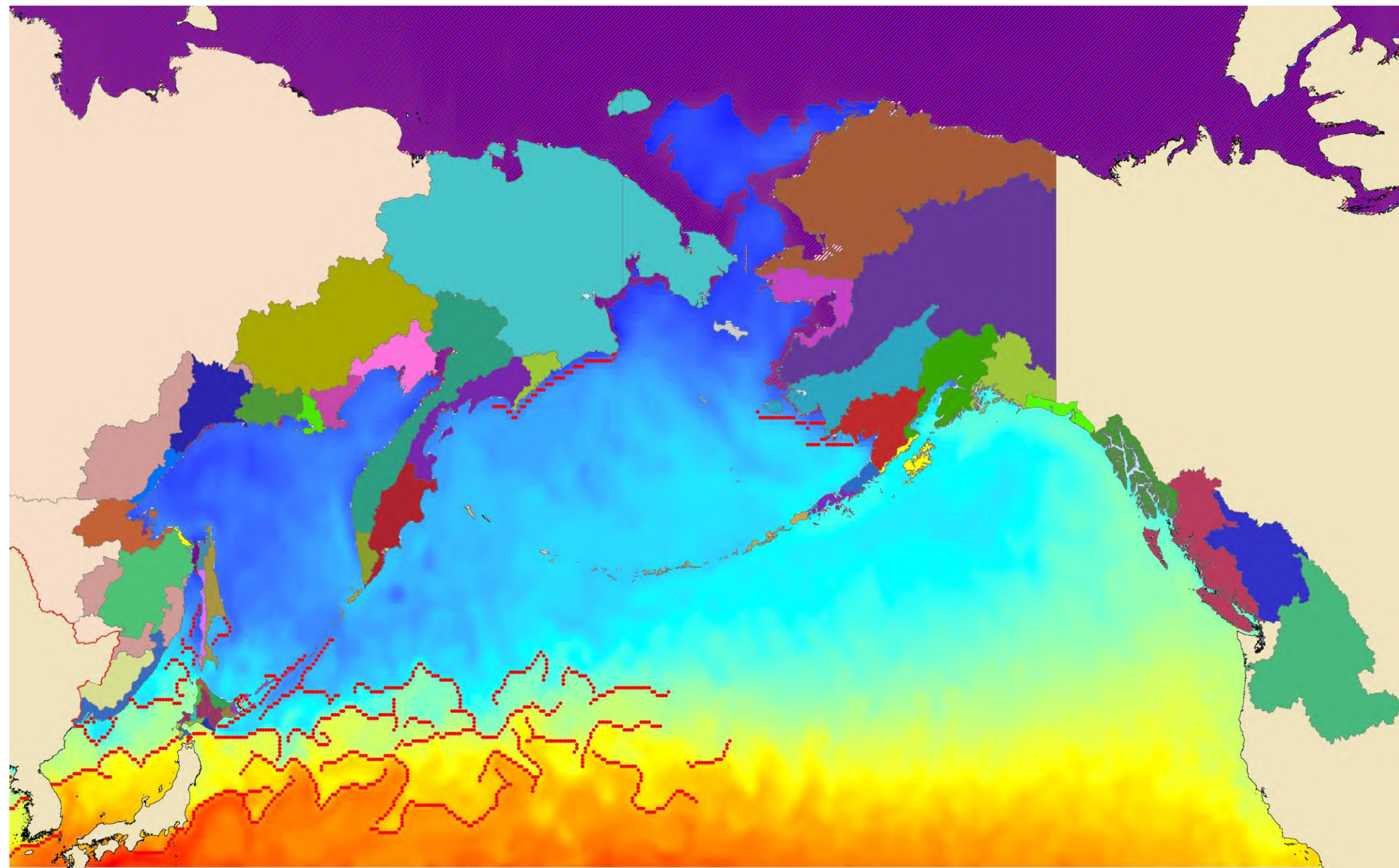
Фронтальные зоны (градиент 1^{\circ}\text{C} и более) на 19 ноября 2025 года
